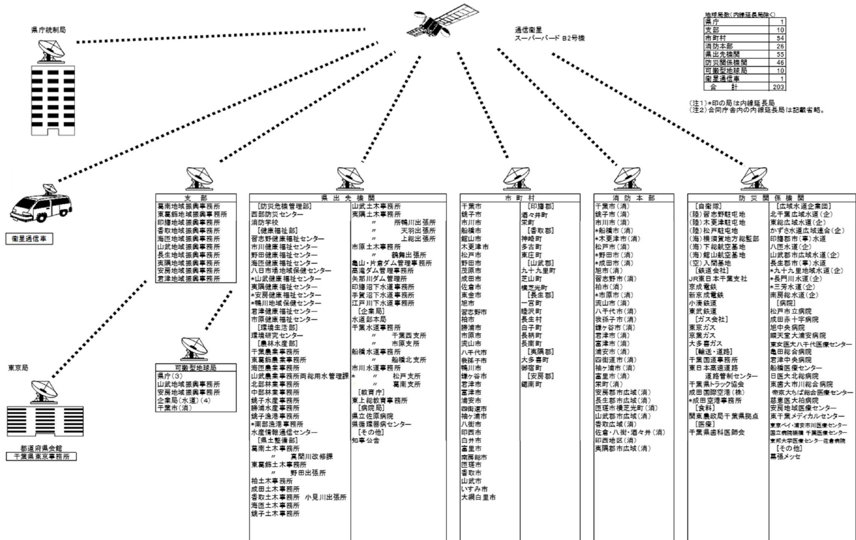
(2) 防災行政無線衛星系回線構成図 (令和3年4月現在)
