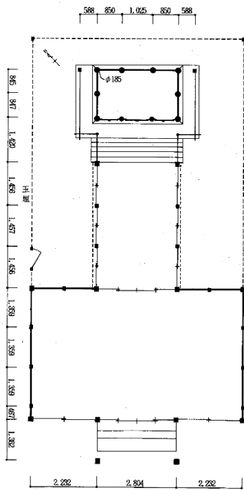
④本殿・拝幣殿平面図
