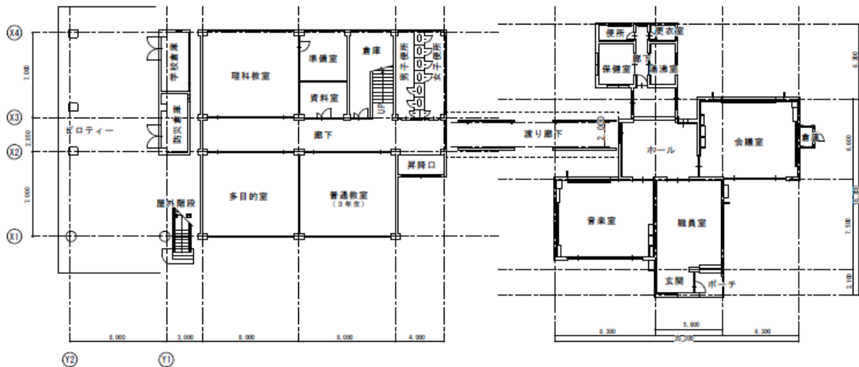
1階平面図
